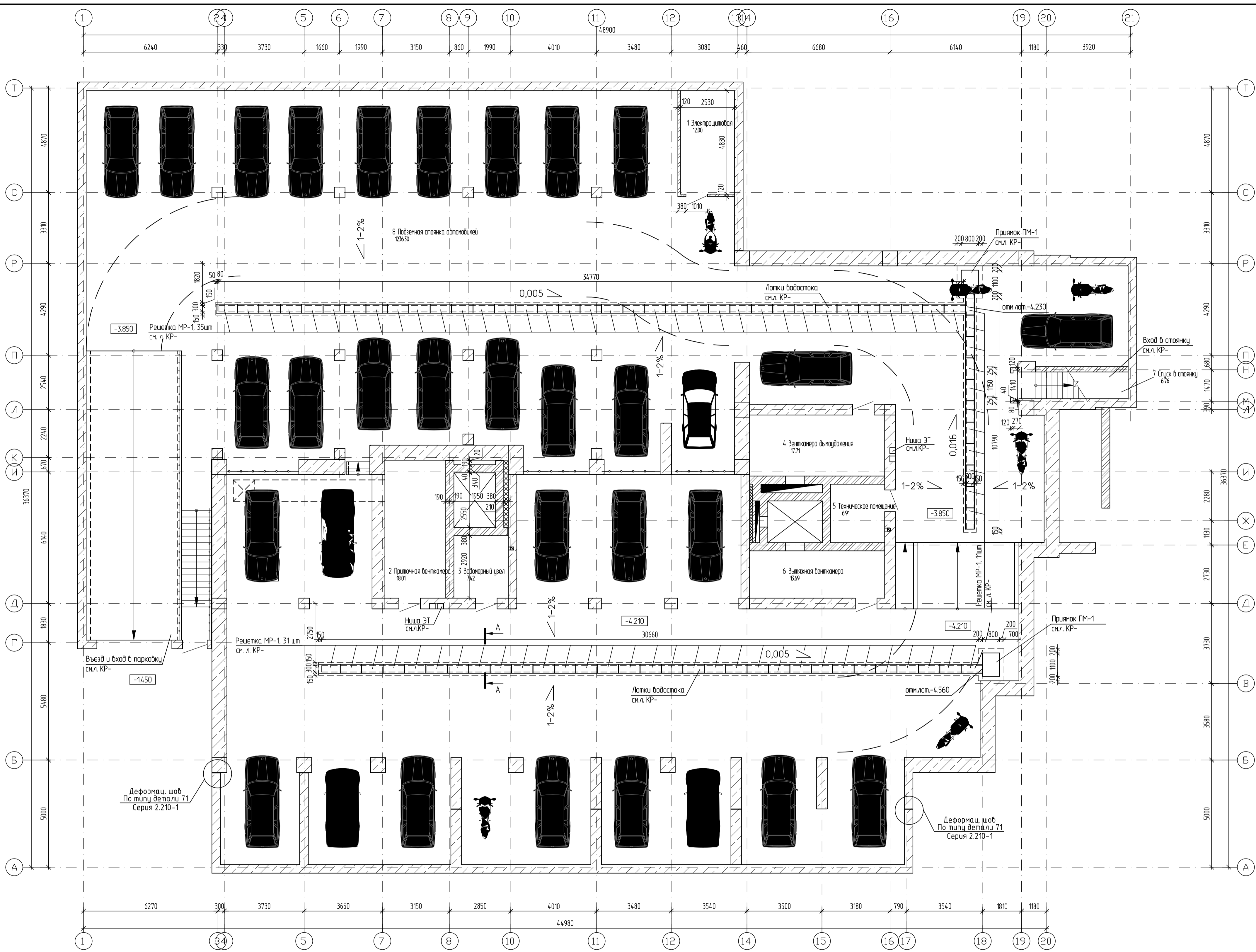
ЭКСПЛИКАЦИЯ ПОМЕЩЕНИЙ
